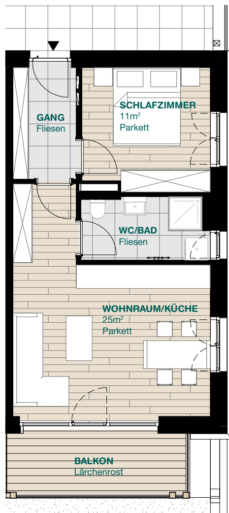
TOP 10 2.OG M 1:100
