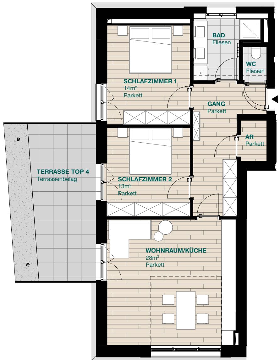
TOP 4 2.OG M 1:100
