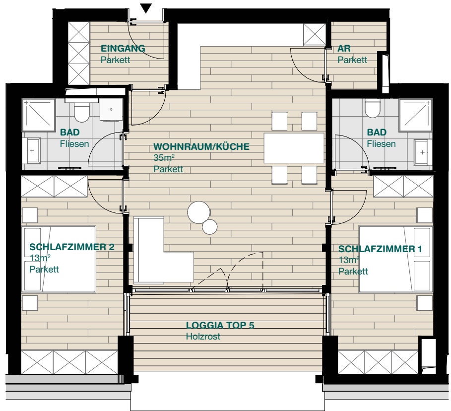
TOP 5 2.OG M 1:100
