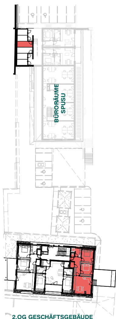
2.OG GESCHÄFTSGEBÄUDE
