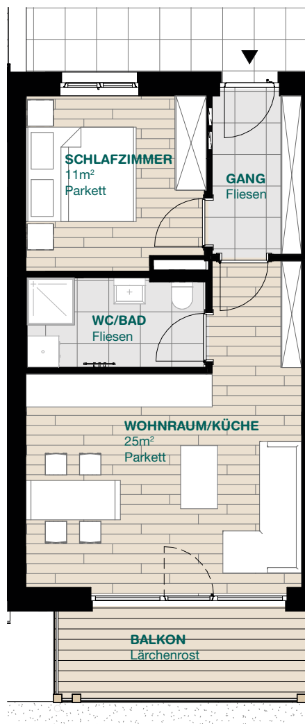
TOP 7 1.OG M 1:100
