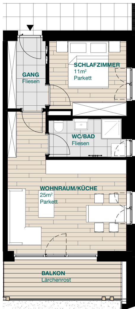
TOP 8 1.OG M 1:100
