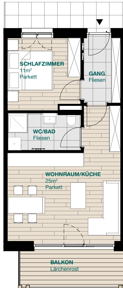
TOP 9 2.OG M 1:100
