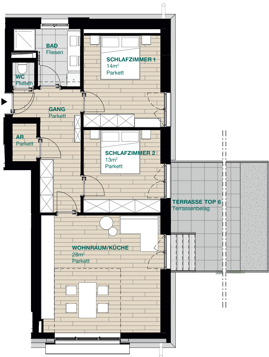
TOP 6 2.OG M 1:100
